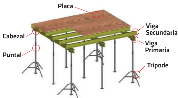
Tripode Plegable Estructura estable, resistente y segura posee un gancho que se ajusta a cualquier puntal. Es plegable lo que permite mayor comodidad en traslado y bodegaje.
